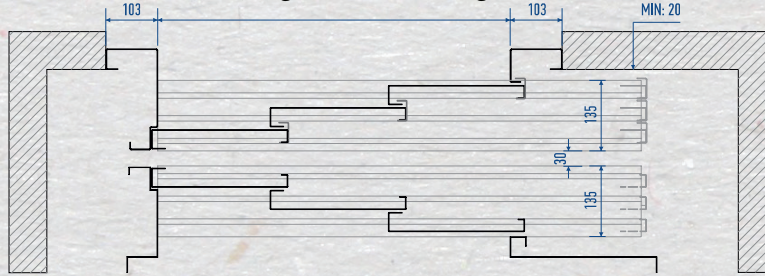
Net Giriş Açıklığı / Clear Opening / ЧИСТЫЙ ПРОЕМ
