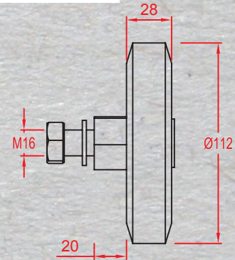
30'luk Makara / 30' Roller / Ролик башмака лифта №30
