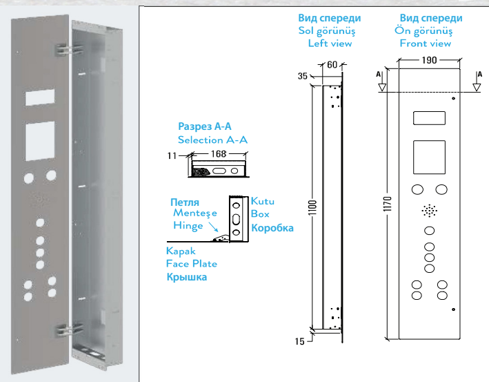
Menteşeli yarım panel / Hinged half C.O.P. / Накладная полуразмерная панель
