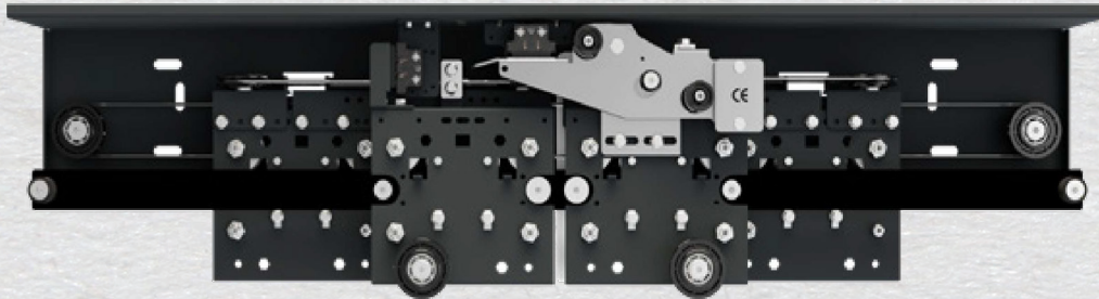
Net Giriş Açıklığı / Clear Opening / ЧИСТЫЙ ПРОЕМ
