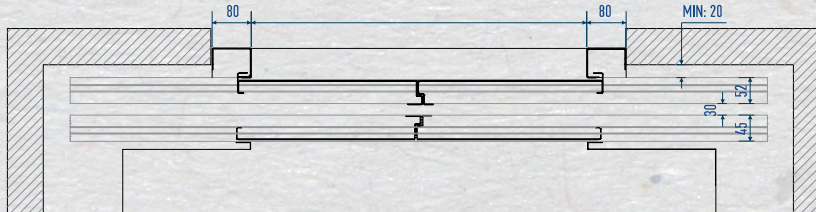
Net Giriş Açıklığı / Clear Opening / Чистый проем
