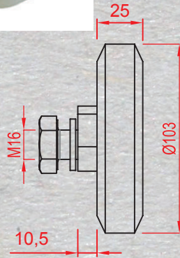
25'lik Makara / 25' Roller / Ролик башмака лифта №25
