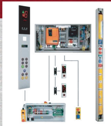
MRL Slim Pano MRL SlimControl Unit Панель MRL Slim
