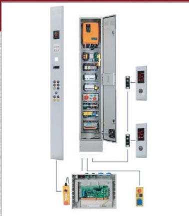
MRL Pano MRL Control Unit Панель MRL
