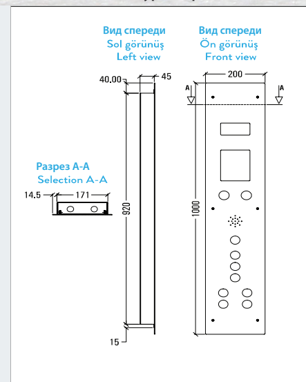
Yaprak kutulu yarım panel / Flush mounted half C.O.P. Утопленная полуразмерная панель
