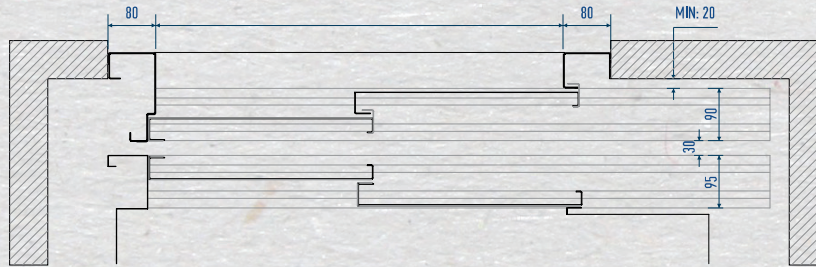
Net Giriş Açıklığı / Clear Opening / Чистый проем
