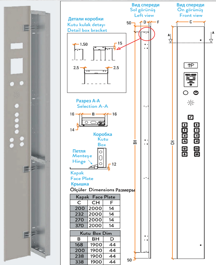
Menteşeli boy panel / Hinged C.O.P. / Накладная полноразмерная панель
