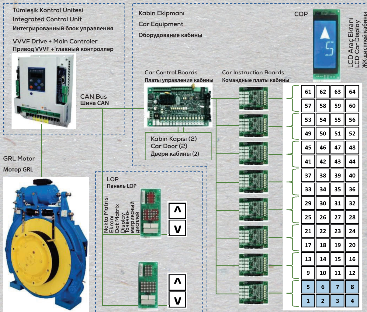
MRL Pano MRL Control Unit Панель MRL
