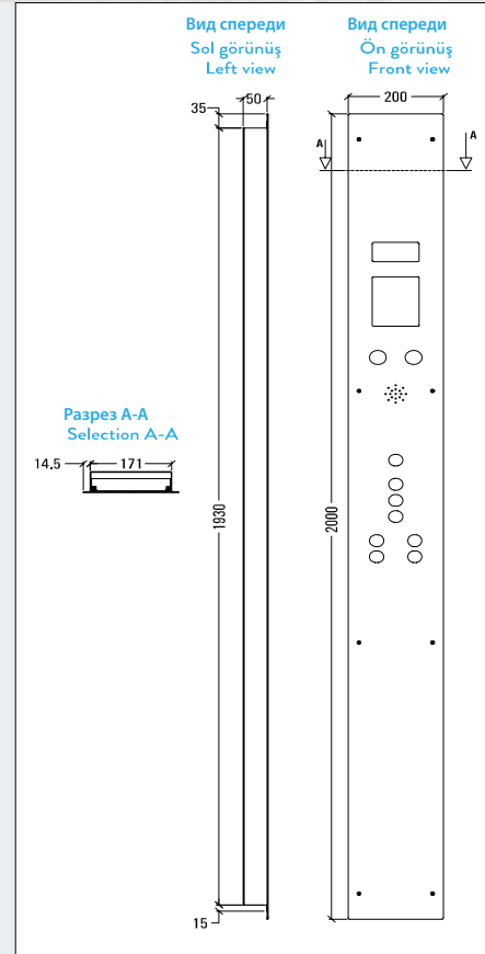
Yaprak kutulu yarım panel / Flush mounted half C.O.P. Утопленная полуразмерная панель
